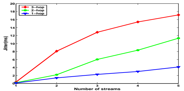
(d) Jitter.
